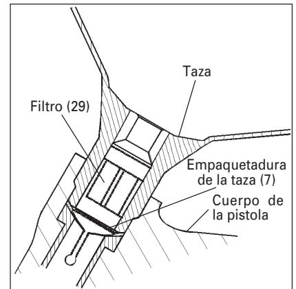
Dibujo de la taza
